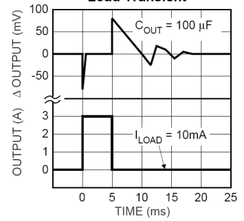
D2632 Load Transient
